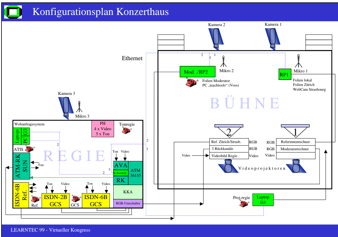
Bild 8: Konfigurationsplan Konzerthaus
