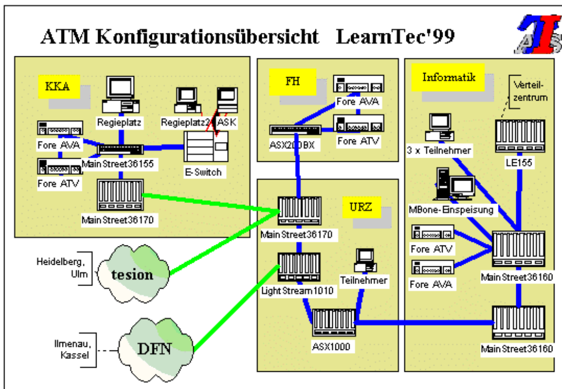
Bild 10: ATM-Verteilung 1999
